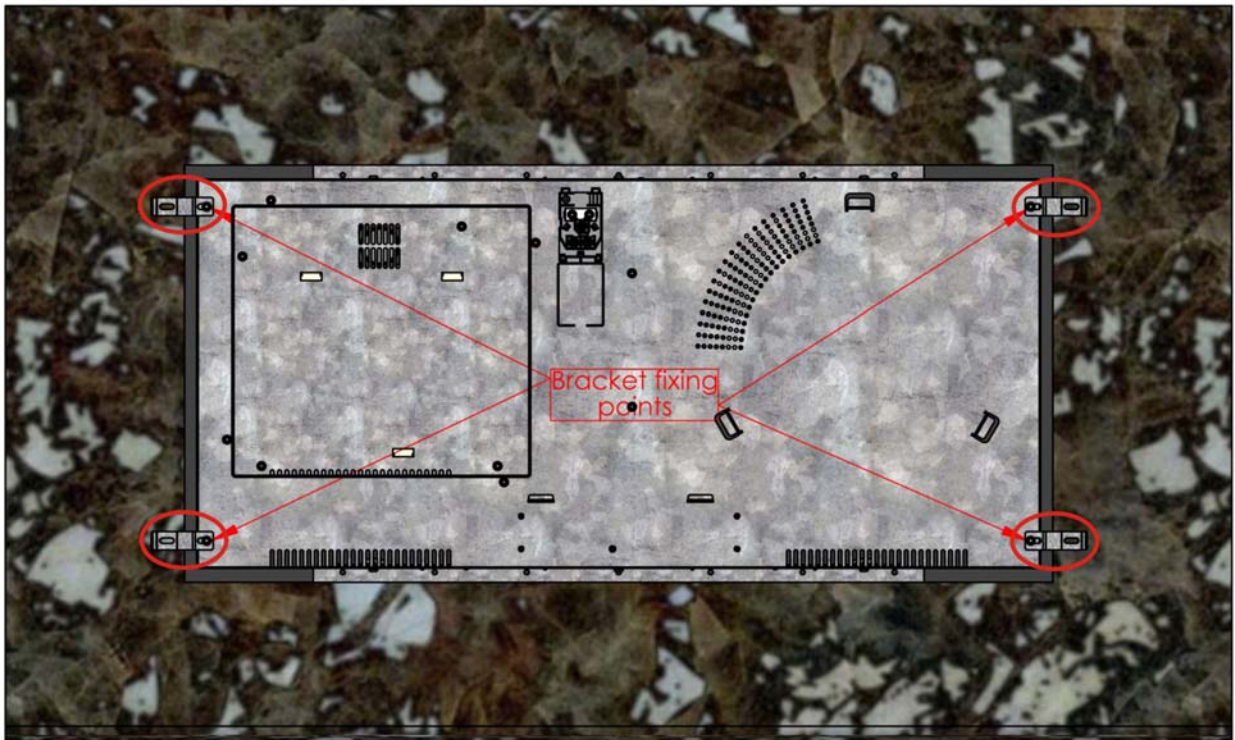
Vị trí lắp pas cố định bếp trên mặt đá
